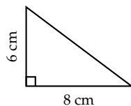
Gambar 1. Segitiga siku-siku
