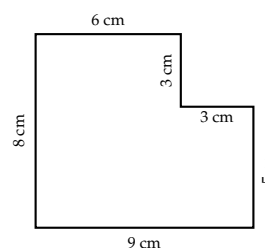
Gambar 10. Bangun datar gabungan
