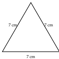
Gambar 3. Segitiga sama sisi
