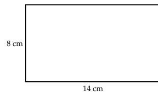
Gambar 2. Persegi panjang PQRS
