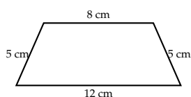
Gambar 8. Trapesium sama kaki
