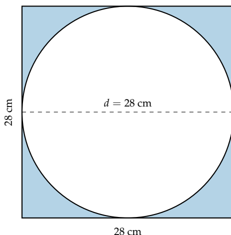
Gambar 1. Persegi dengan lingkaran di dalamnya
