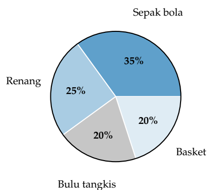
Gambar 2. Kegiatan ekstrakurikuler yang digemari 120 siswa
