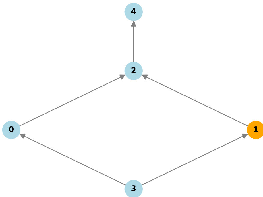
Poset
