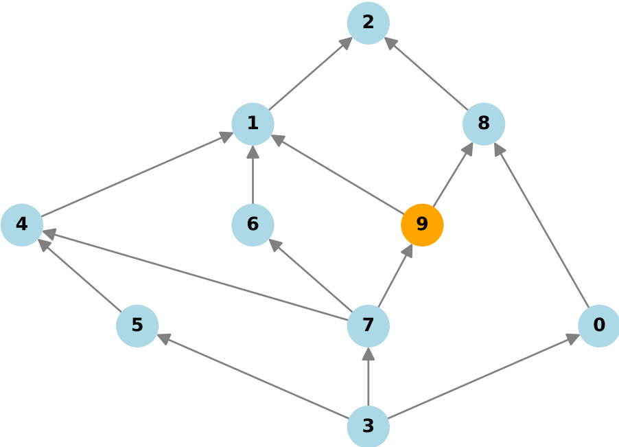
Poset
