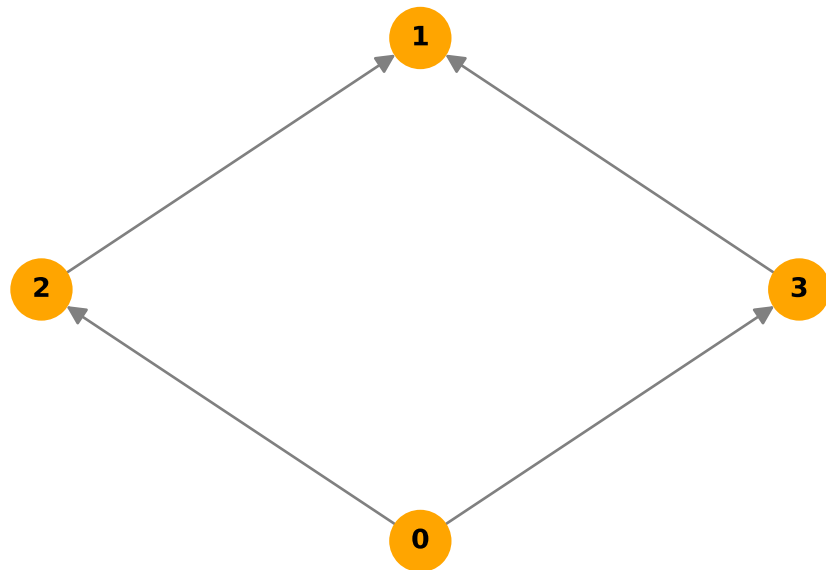
Poset
