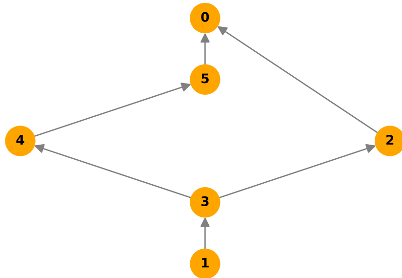
Poset
