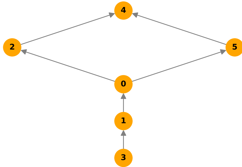
Poset
