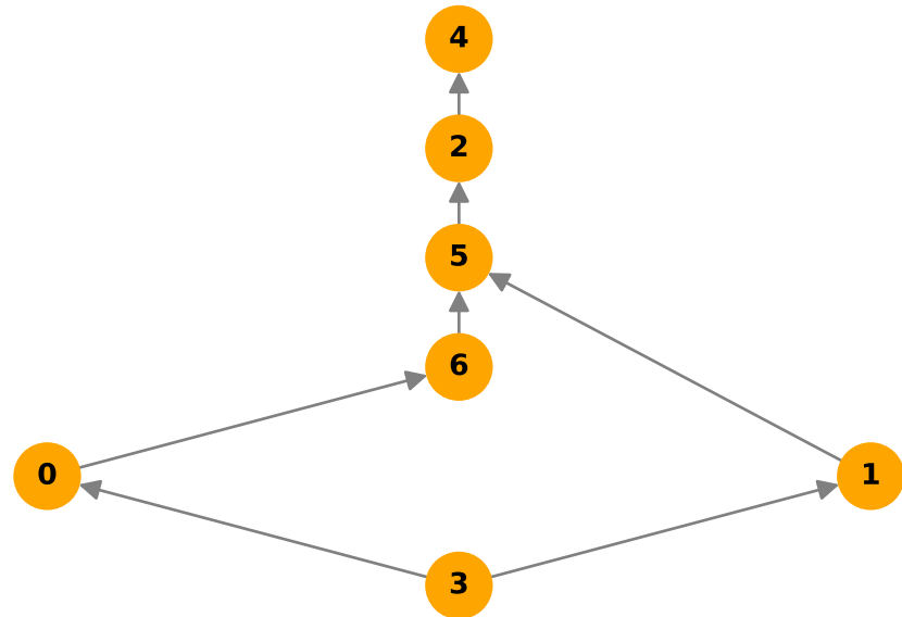
Poset
