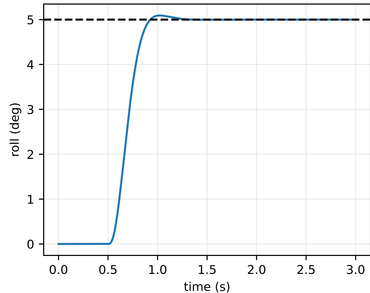
5° roll step
