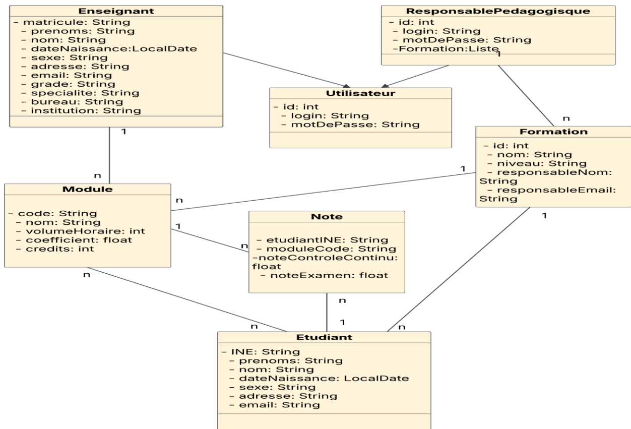
Figure 1: Diagramme de classe du projet
