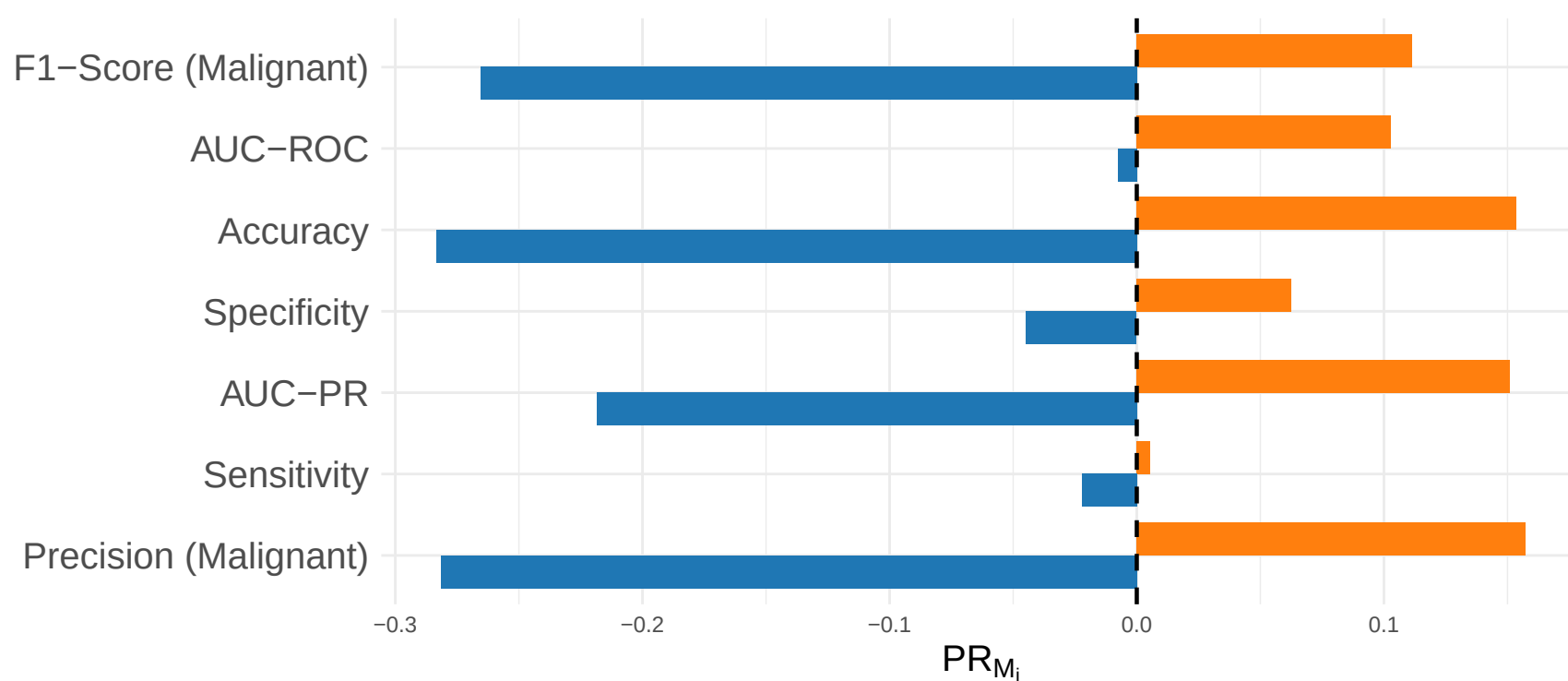
VGG16
