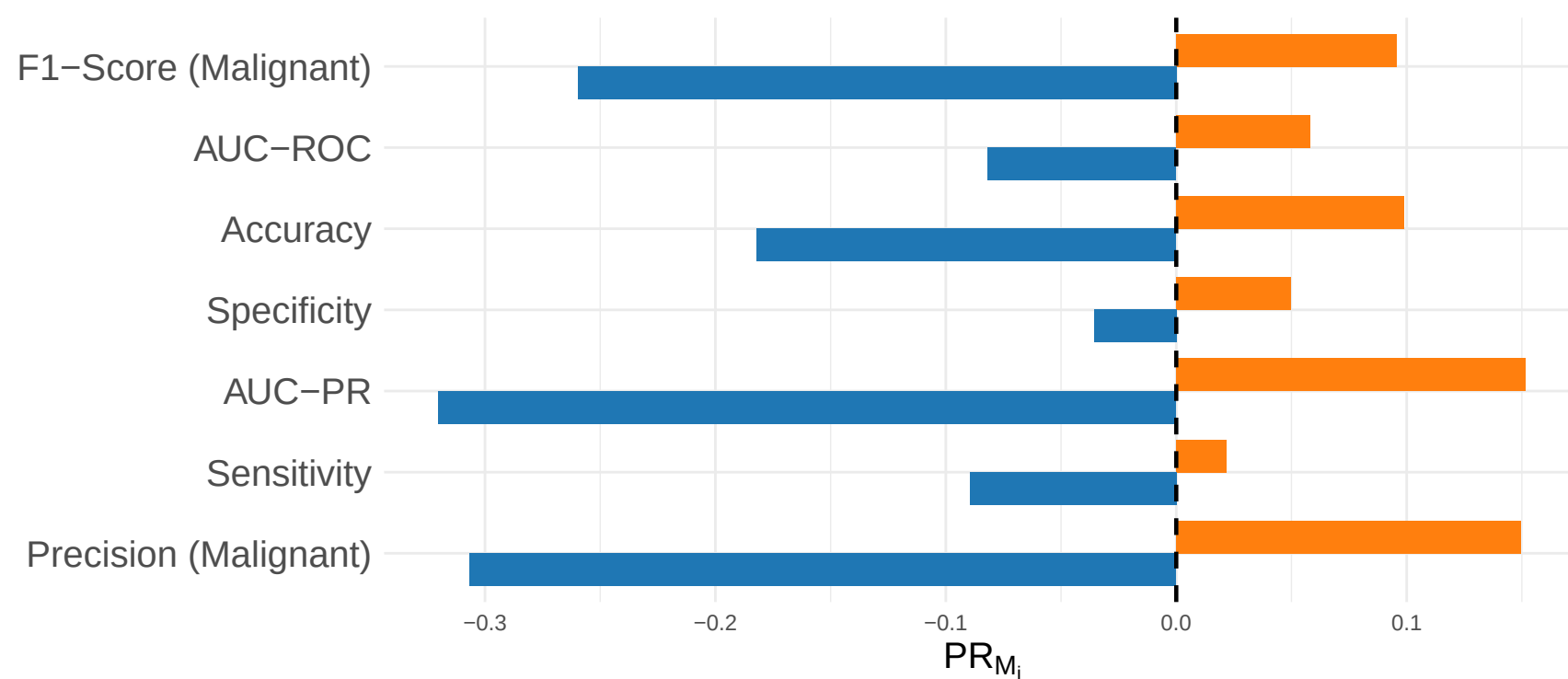
EfficientNetV2B0
