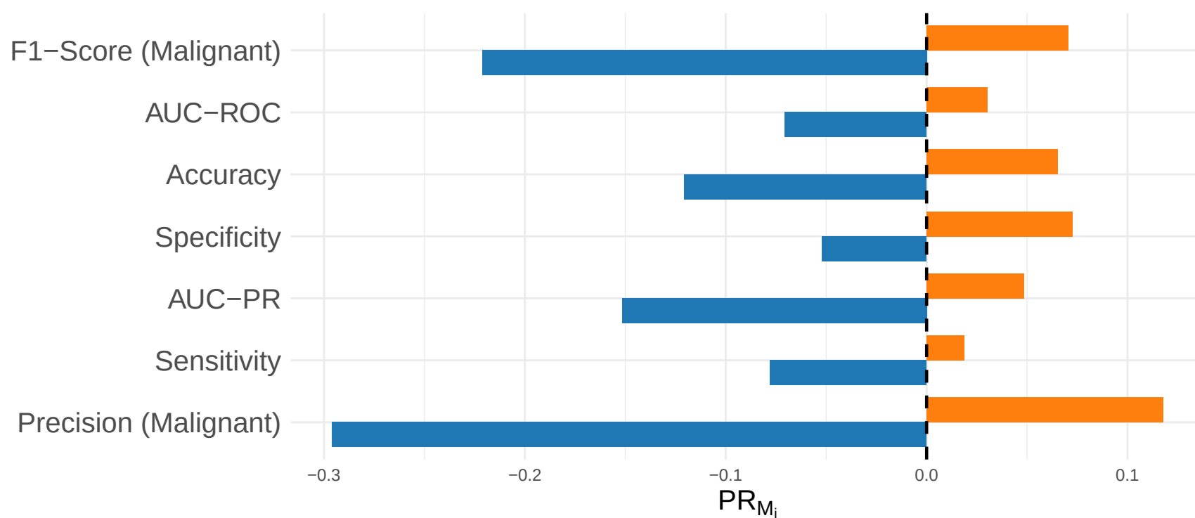
MobileNetV2
