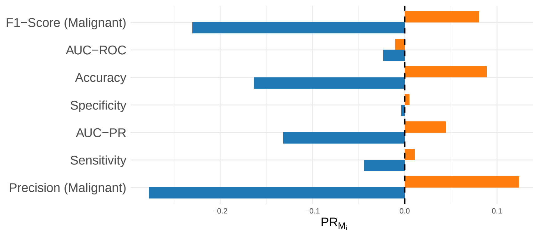
EfficientNetV2B0
