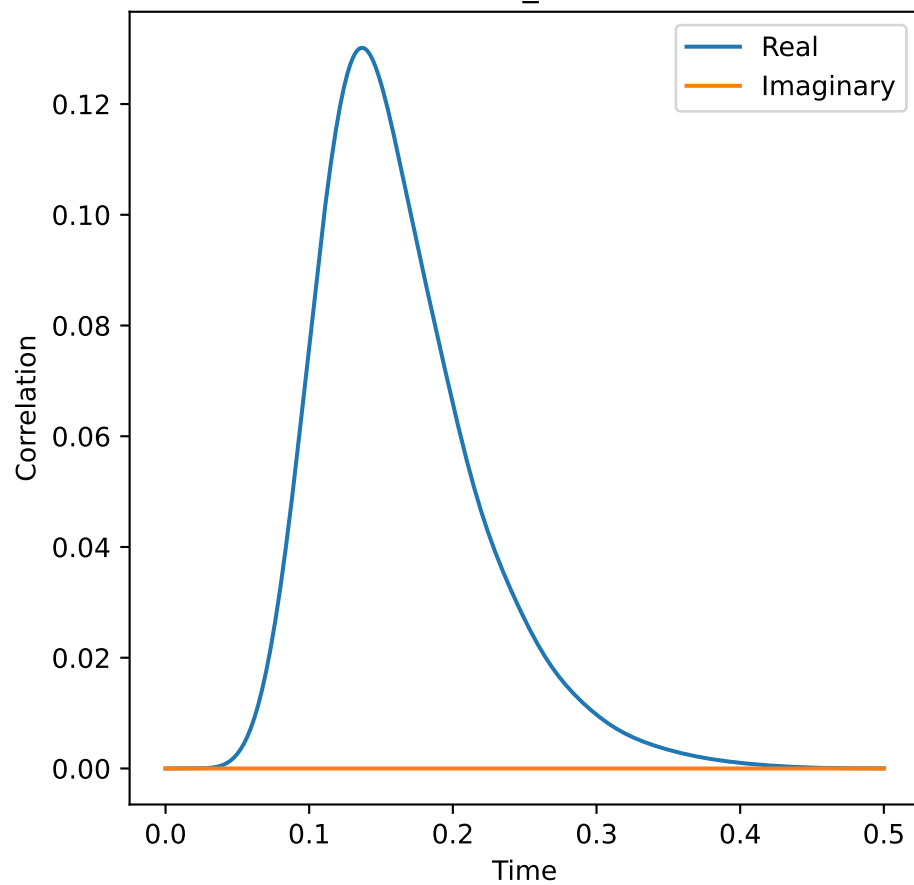
rho_10
