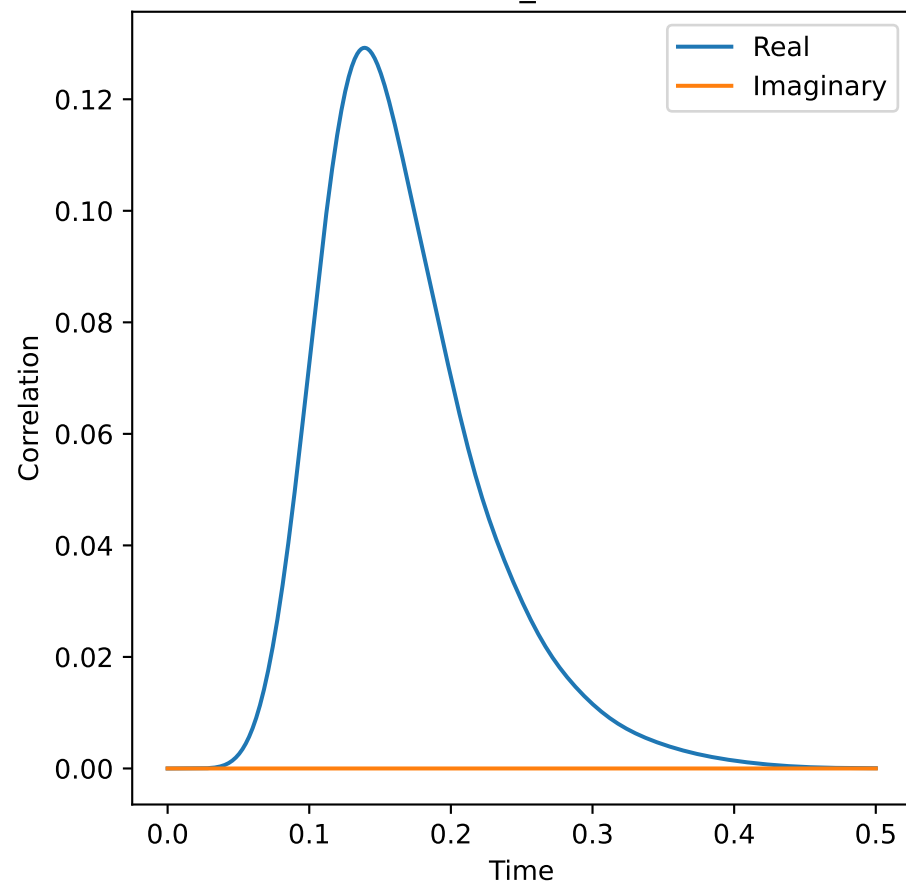
rho_01
