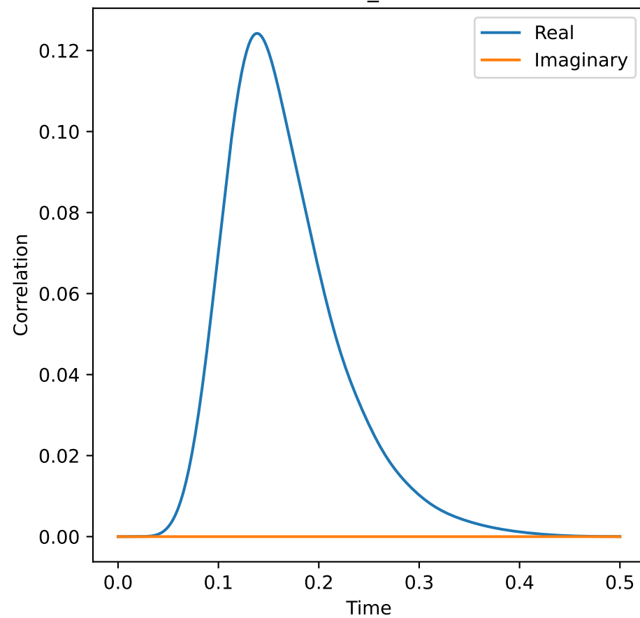
rho_01
