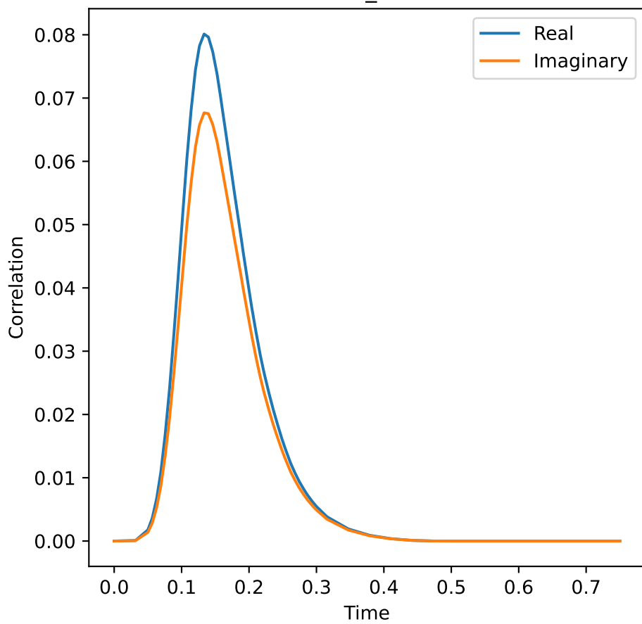
rho_10
