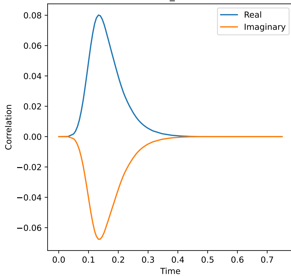
rho_01
