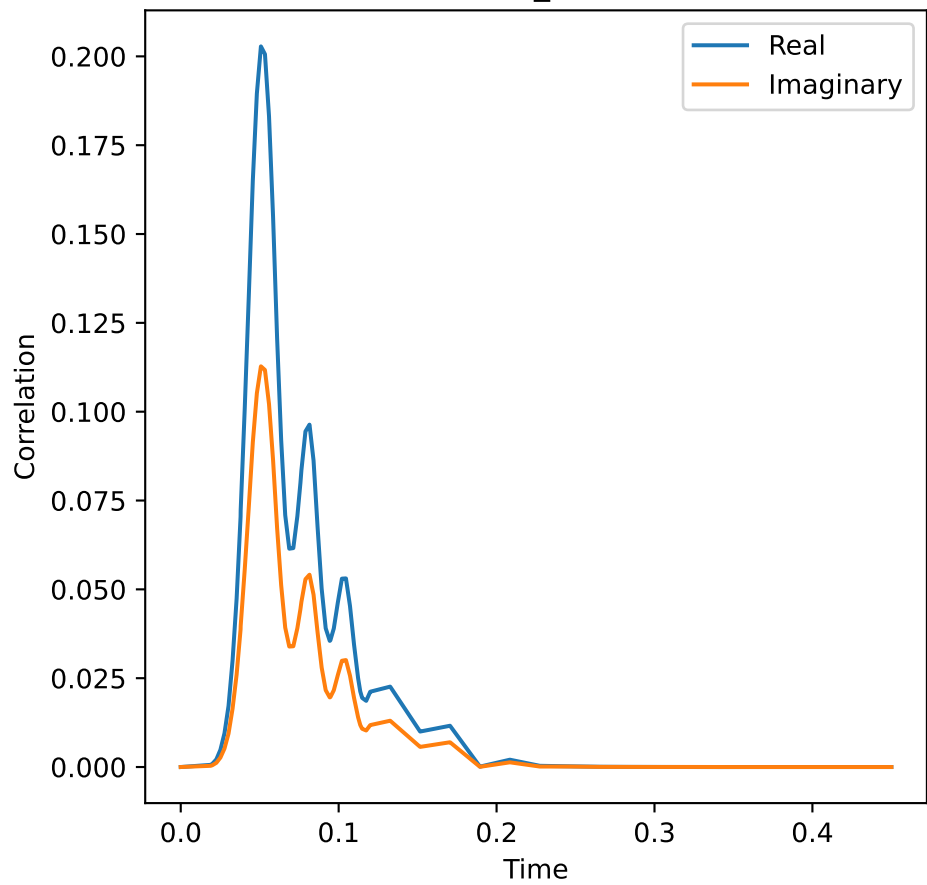
rho_10
