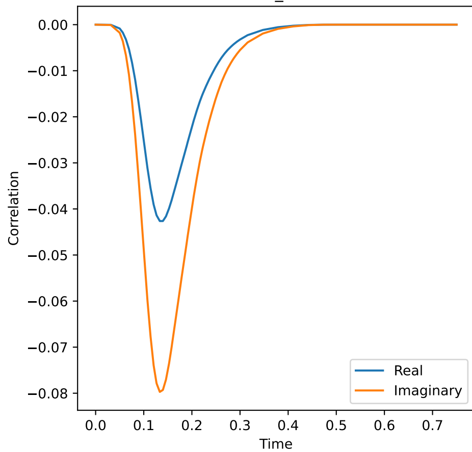
rho_01
