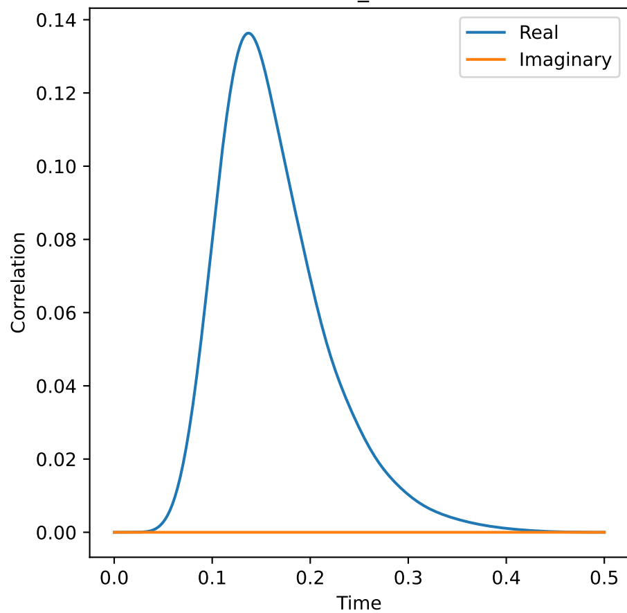
rho_10
