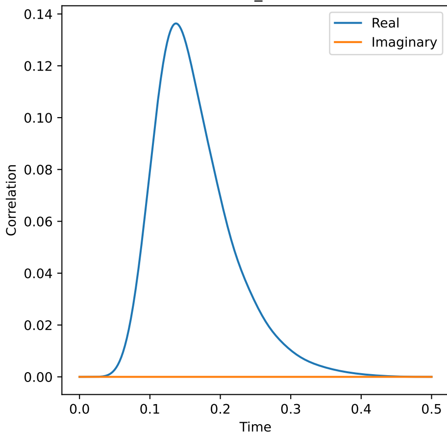
rho_10
