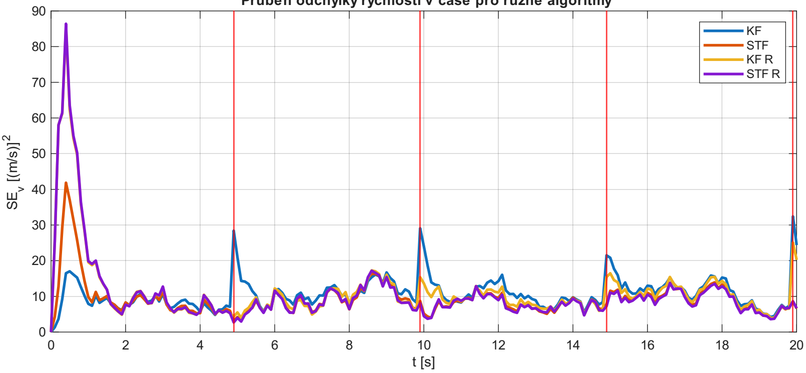
Průběh odchylky rychlosti v čase pro různé algoritmy
