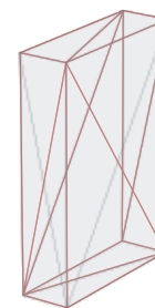
V-HACD
