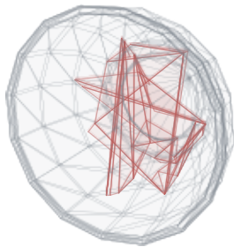
V-HACD package
