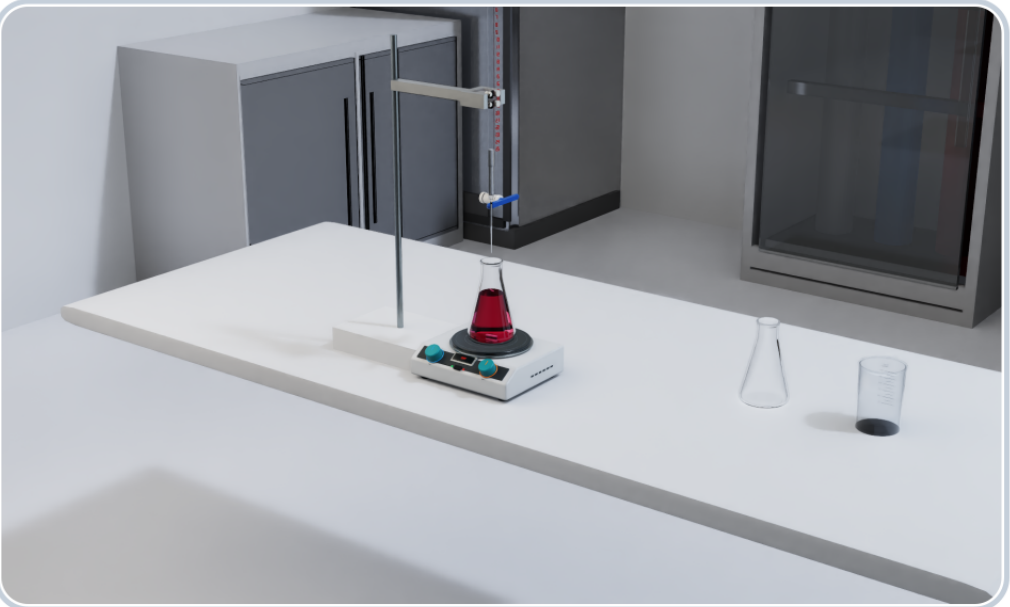
Titration
