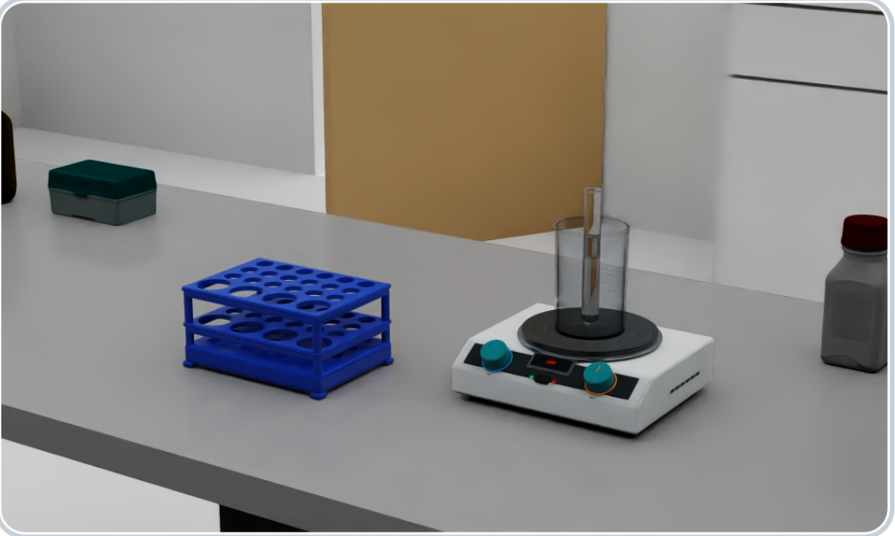
Fehling
