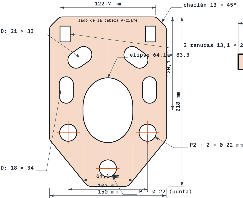
05 • ALA (ESCUDO) • FABRICAR × 1 ESCALA 1:2,31
