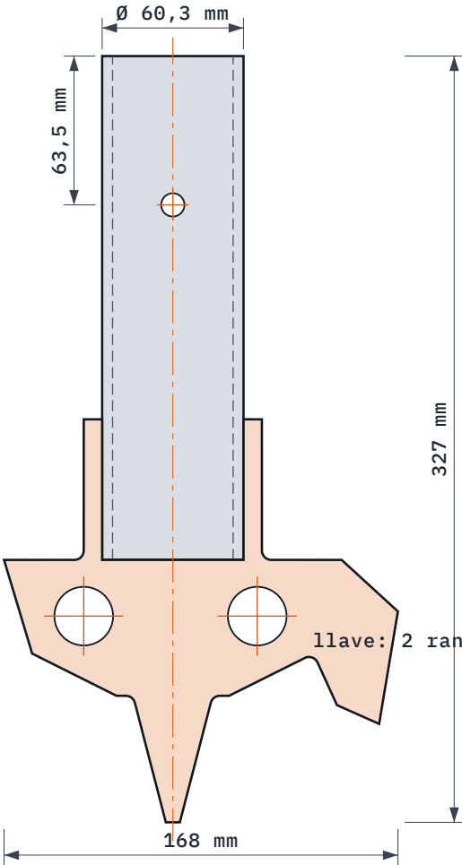
14 · PIE DE FLECHA · FABRICAR × 3 ESCALA 1:2,89
