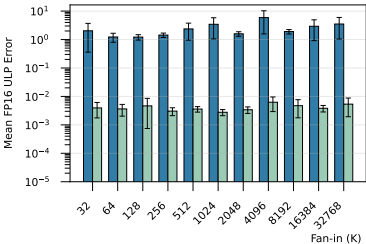
FP16-INT4 QCOL
