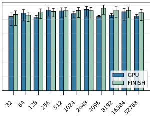
FP16-INT4 QROW
