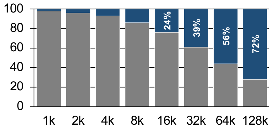
Llama-3 70B
