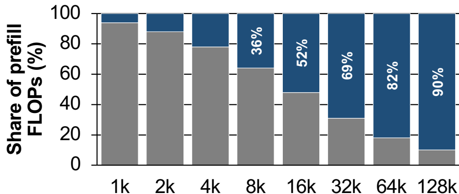
Llama-3 8B
