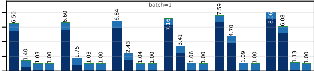
llama3 Prefill
