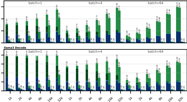
llama2 Decode
