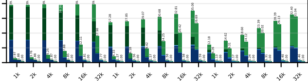
llama3 Decode
