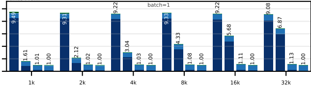
llama2 Decode
