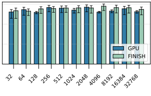
FP16-INT4 QROW
