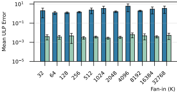
FP16-INT4 QCOL
