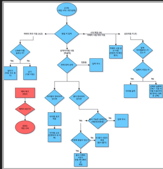
플레이어의 기능에 대한 플로우 차트
