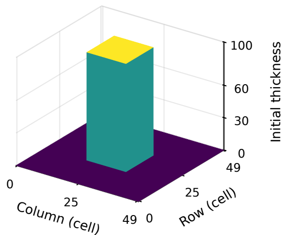
(d) Center-100
