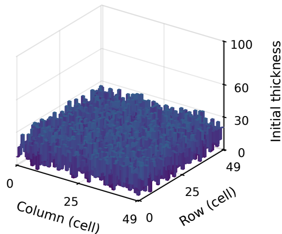
(d) Center-100
