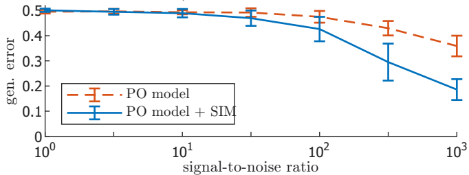
a) Generalisation error
