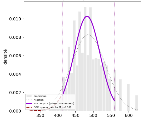
Figure 9 — Diagnostics de distributions globales ( Y et M ) : histogrammes, ajustement gaussien du corps, et ajustements de queues lourdes sur les extrêmes (modélisation type GPD) avec paramètre d'exposant de queue \xi ( ksi ).
