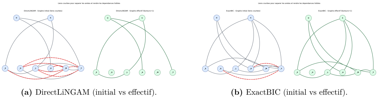
Figure 7 – Graphes causaux utilisés dans STAR (visualisation des structures initiales et effectives).
