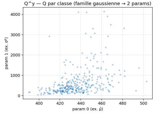
(b) Distribution enrichie de Q^y (DirectLiNGAM, \text{do}(1) ).
