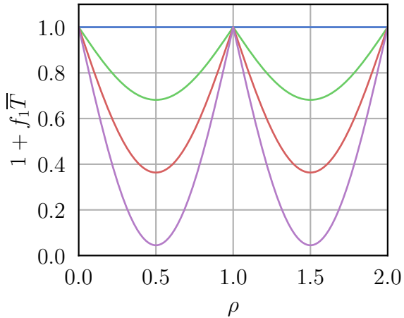
(d) U = 3W/2
