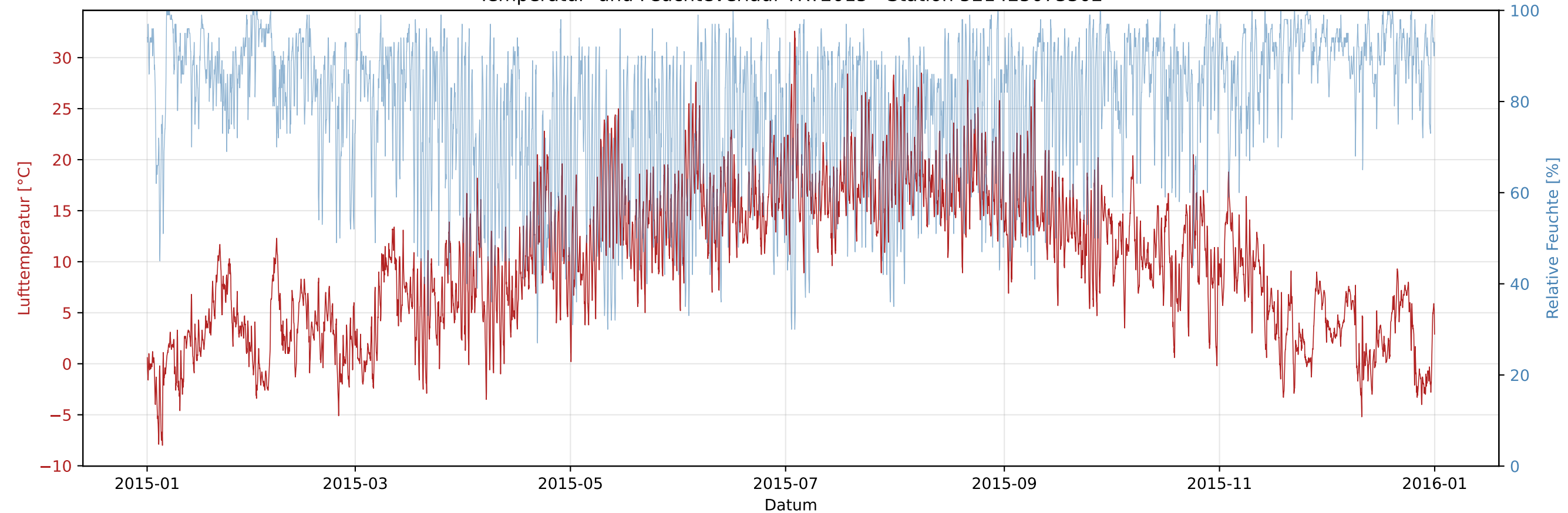
Temperatur- und Feuchteverlauf TRY2015 - Station 521425073302
