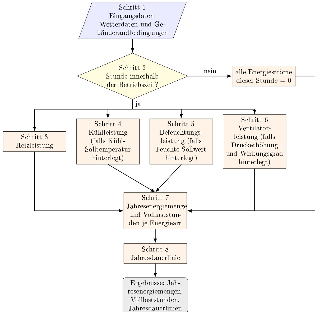
Abbildung 3.1.: Ablauf der stündlichen Berechnung der Lüftungsenergieströme
