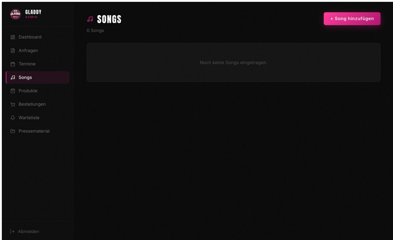
Abb. 5.1 — Songs-Verwaltung
