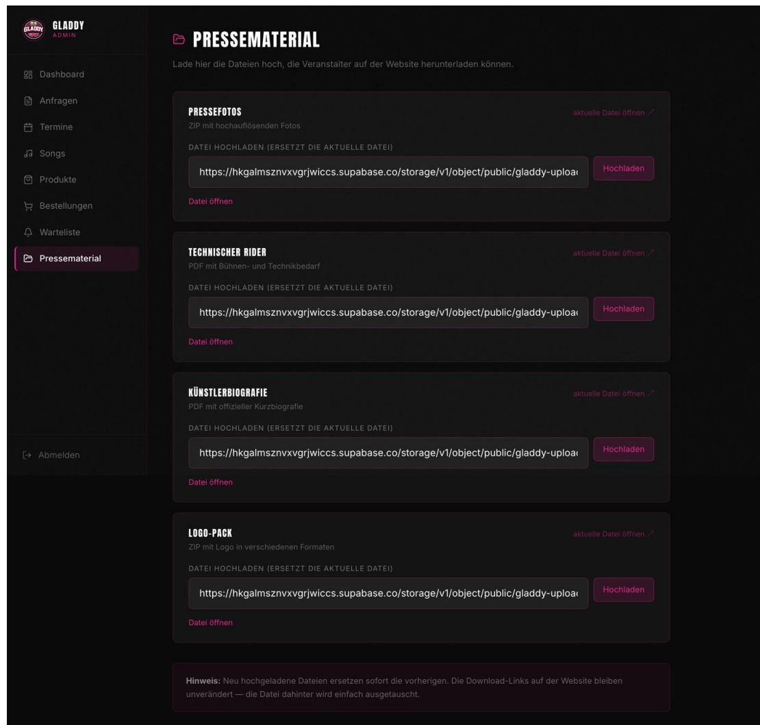
Abb. 9.1 — Pressematerial-Verwaltung
