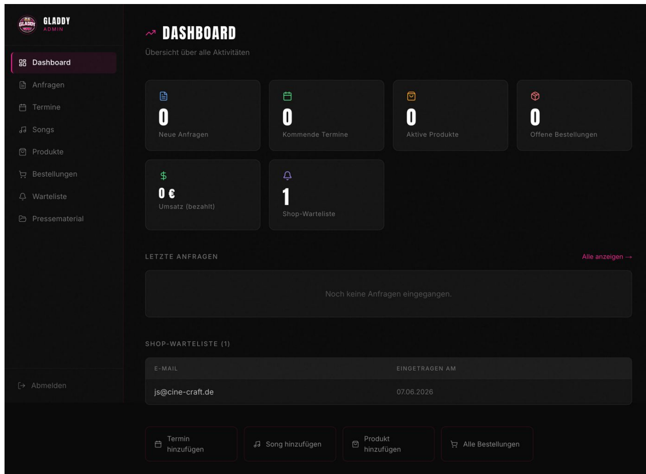
Abb. 2.1 — Dashboard Übersicht
