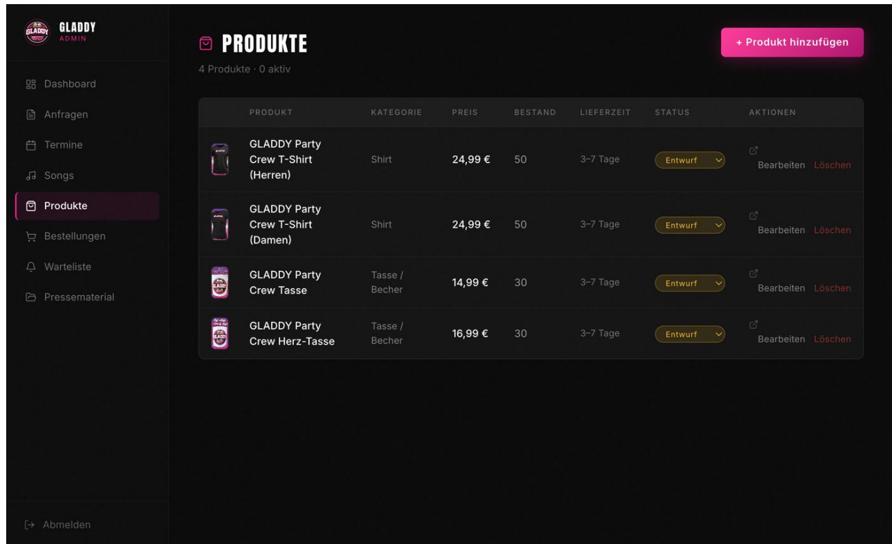
Abb. 6.1 — Produkte-Liste
