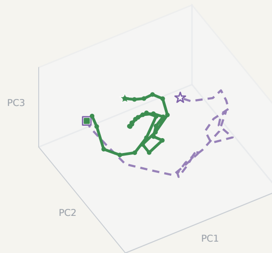
LeWM + CGS
