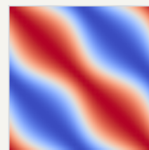
LeWM + TS
