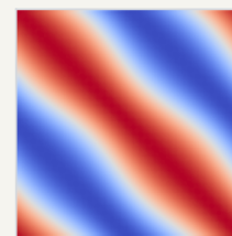
LeWM + CGS
