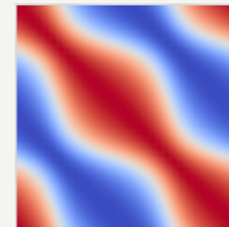
LeWM + CGS
