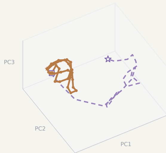
LeWM + TS
