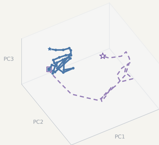
LeWM
