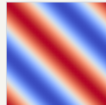
LeWM + TS
