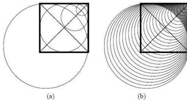
图 7.2.5 用圆的并集重建区域
