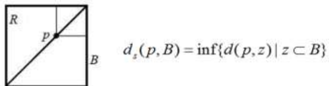
图 7.2.3 区域 R ，边界 B 和骨架点 P
