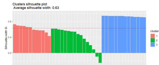
(b) Gráfico de Silhouette
