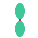
p (แสดงแกน x) p (แสดงแกน y) ต้มเบสสองพู่ วางตาม 3 แกนตั้งฉาก (x, y, z) \rightarrow ชั้นเซลล์ 3 ออร์บิทัล
