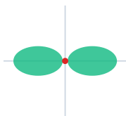
p (แสดงแกน x) p (แสดงแกน y) ต้มเบสสองพู่ วางตาม 3 แกนตั้งฉาก (x, y, z) \rightarrow ชั้นเซลล์ 3 ออร์บิทัล
