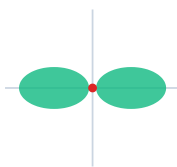
p (แสดงแกน x) p (แสดงแกน y) ดัมเบลสองพู วางตาม 3 แกนตั้งฉาก (x, y, z) \rightarrow ชั้นเซลล์ 3 ออร์บิทัล
