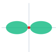
p (แสดงแกน x) p (แสดงแกน y) ต้มเบลสองพู่ วางตาม 3 แกนตั้งฉาก (x, y, z) \rightarrow ชั้นเซลล์ 3 ออร์บิทัล
