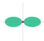
p (แสดงแกน x) p (แสดงแกน y) ตั้มเบลสองพู วางตาม 3 แกนตั้งฉาก (x, y, z) → ขับเชลล์ล 3 ออร์บิทัล
