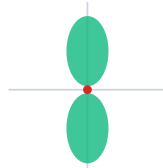
p (แสดงแกน x) p (แสดงแกน y) ตั้มเบลสองพู วางตาม 3 แกนตั้งฉาก (x, y, z) → ขับเชลล์ล 3 ออร์บิทัล
