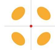
d (ตัวอย่าง 1 ใน 5 แบบ) ส่วนใหญ่เป็นไบโโคเวอร์ 4 พู ชั้นเซลล์ละ 5 ออร์บิทัล
