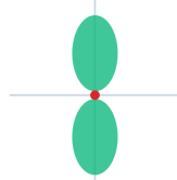
p (แสดงแกน x) p (แสดงแกน y) ตั้มเบลสองพู วางตาม 3 แกนตั้งฉาก (x, y, z) → ขับเชลล์ล 3 ออร์บิทัล
