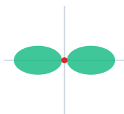
p (แสดงแกน x) p (แสดงแกน y) ตั้มเบลสองพู วางตาม 3 แกนตั้งฉาก (x, y, z) → ขับเชลล์ล 3 ออร์บิทัล
