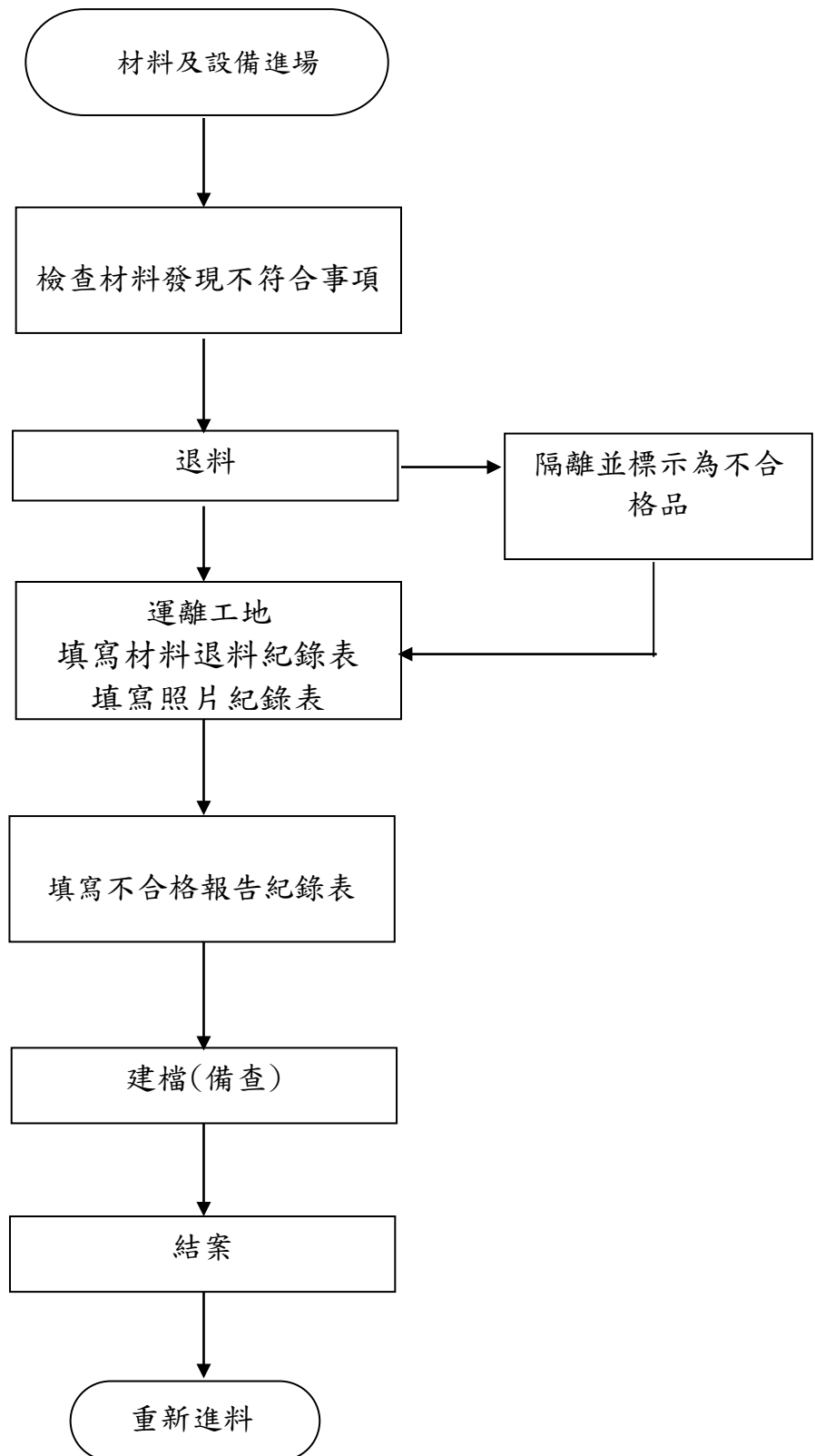
圖 八-1 材料自主檢查不合格管制作業流程
