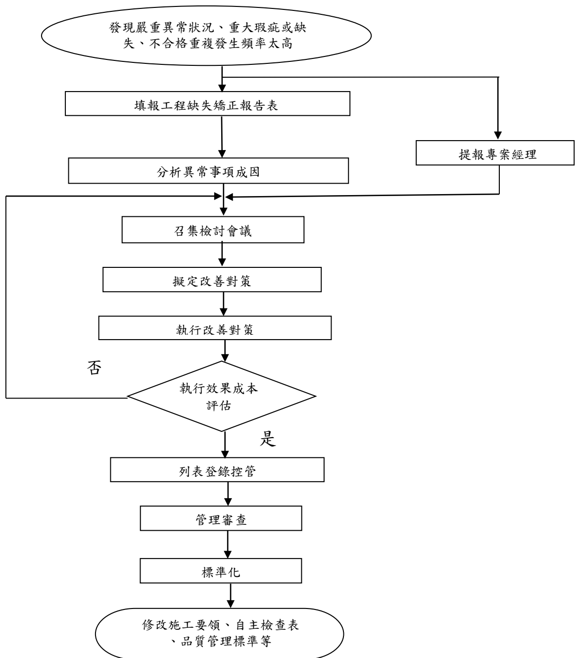
圖 九-1 矯正措施流程圖
