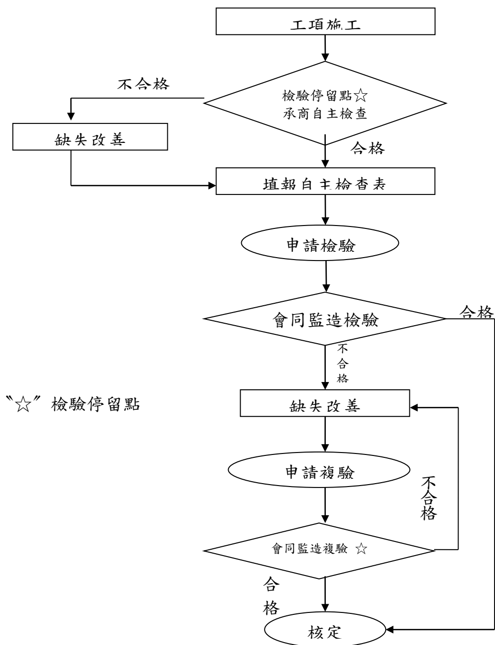
圖 五-2 施工檢驗流程圖
