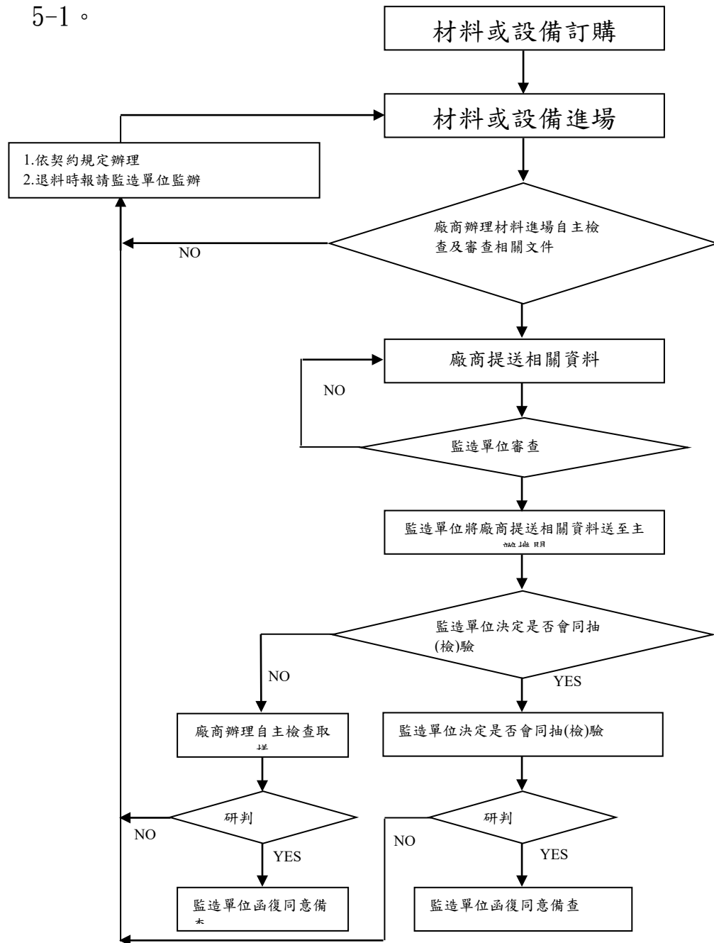
圖 五-1 材料設備檢驗流程圖
