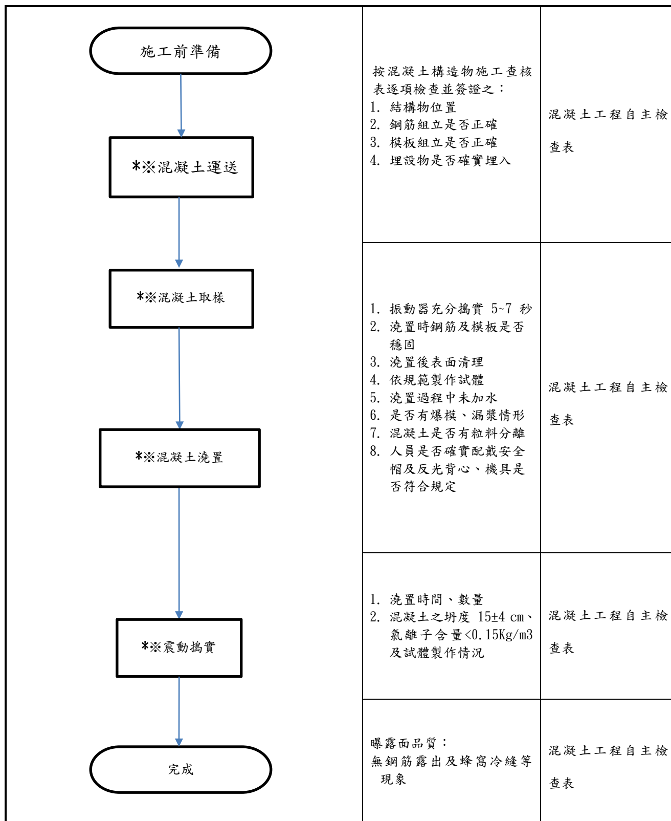
圖 5-7-4、混凝土工程施工作業流程及檢驗圖
