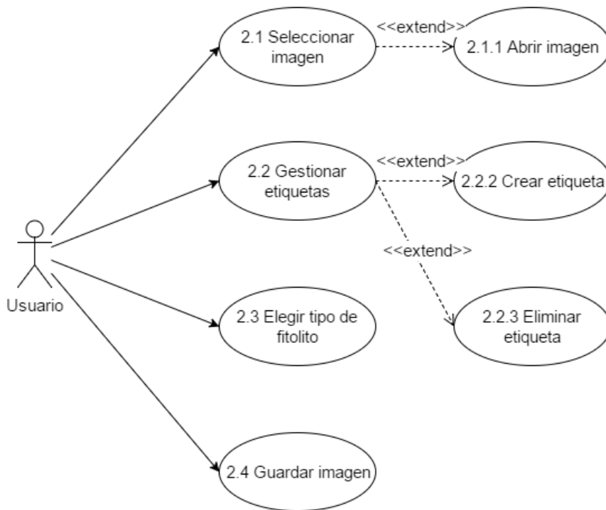
Figura B.2: Diagrama extendido de casos de uso
