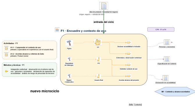
Figura 2. Fragmento SPEM 2.0 de F1: actividades A1.1 y A1.2, sus roles primarios y los productos de trabajo de salida. Cierra con el hito M1 y no tiene compuerta.
