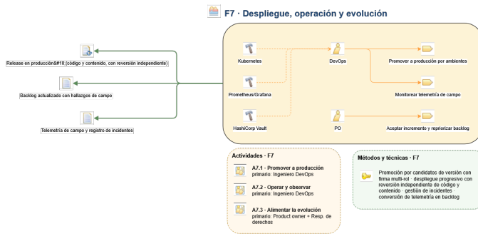
Figura 8. Fragmento SPEM 2.0 de F7: actividades A7.1 a A7.3. La fase no tiene compuerta porque lo desplegado ya superó G1 y G2; la telemetría de campo realimenta el backlog .
