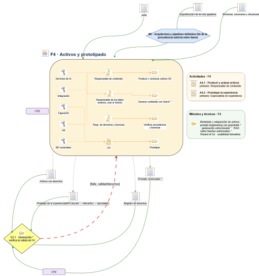
Figura 5. Fragmento SPEM 2.0 de F4: actividades A4.1 y A4.2. La compuerta condicional G3 verifica la procedencia de todo activo antes de su entrada a la cadena de contenido.
