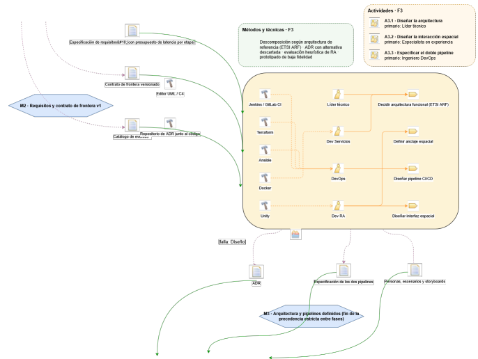
Figura 4. Fragmento SPEM 2.0 de F3: actividades A3.1 a A3.3. El hito M3 cierra la precedencia estricta entre fases; a partir de él el microciclo extrae trabajo de las fases activas.
