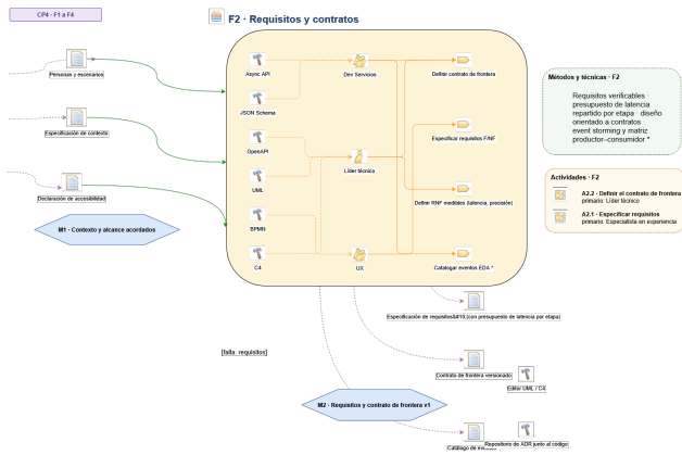
Figura 3. Fragmento SPEM 2.0 de F2: actividades A2.1 y A2.2. El contrato de frontera adopta la forma de contrato de eventos cuando EDA está activo y de esquemas de datos cuando no lo está.
