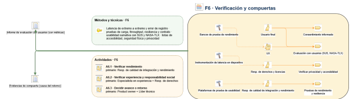
Figura 7. Fragmento SPEM 2.0 de F6: actividades A6.1 a A6.3 y las compuertas G1 y G2. Las flechas de retorno llevan la causa registrada y la fase de destino que prescribe cada compuerta.
