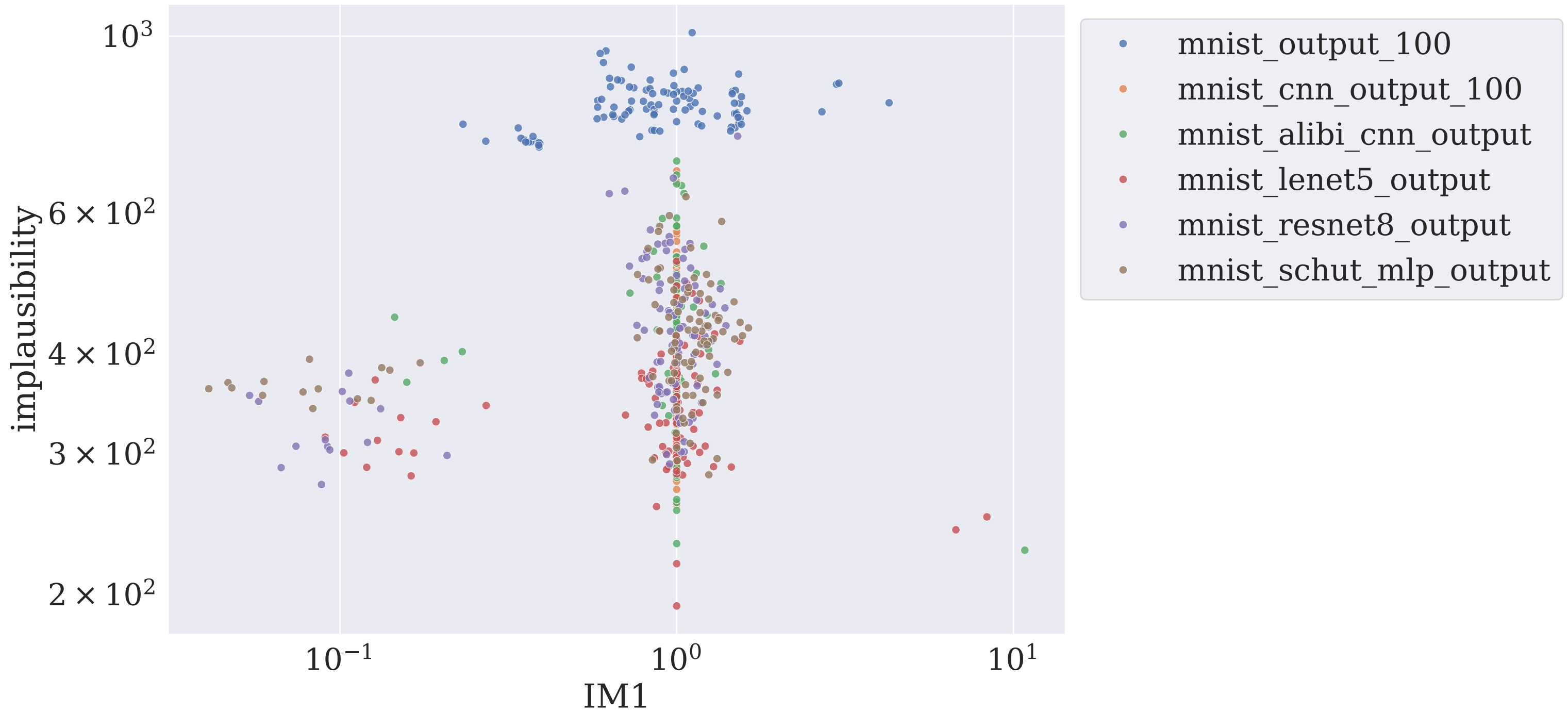
implausibility vs IM1
