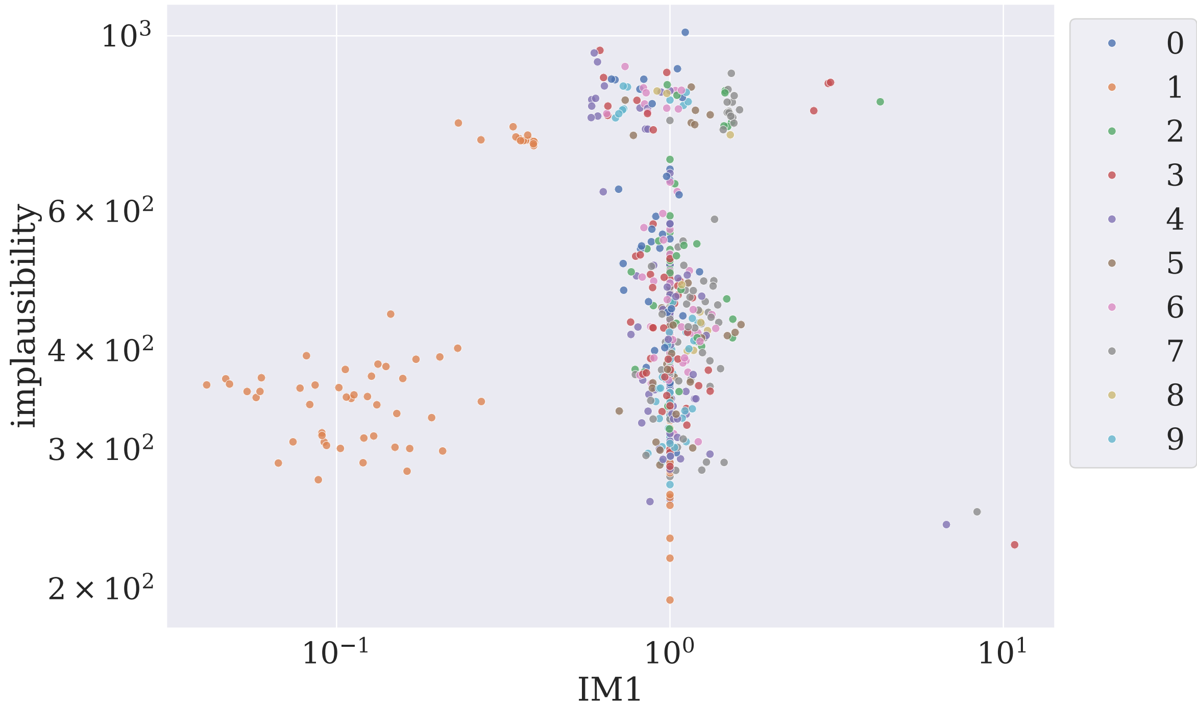
implausibility vs IM1
