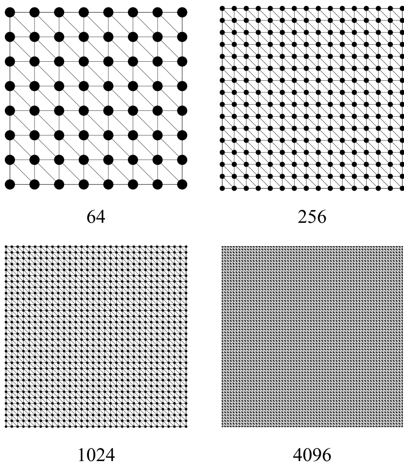
图 4.2 固支方板挠度场的节点布置（图中数字为节点数）
