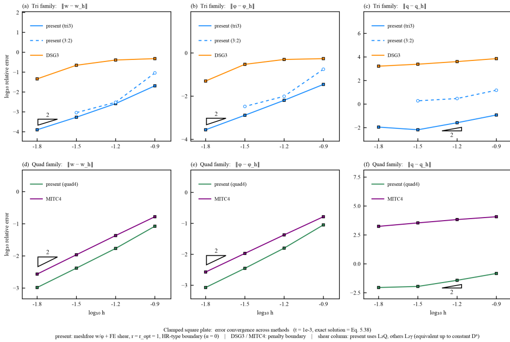
图 4.4 固支方板挠度、转角与剪力的误差收敛对比（上排为三角单元族，下排为四边形单元族）
