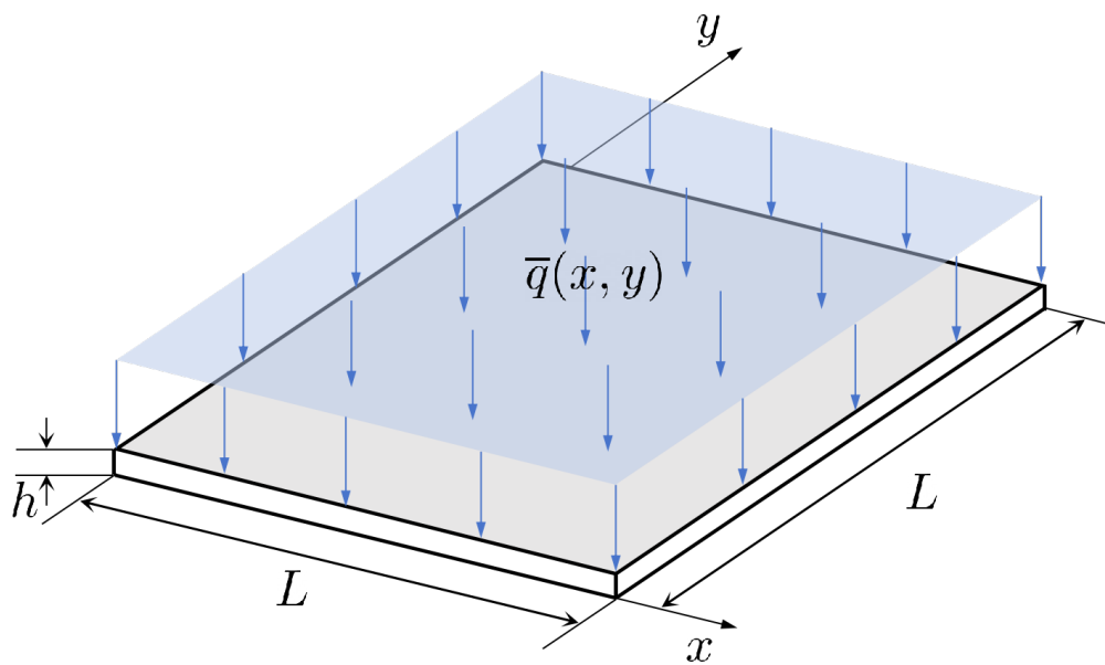
图 4.1 四边固支方板示意图
