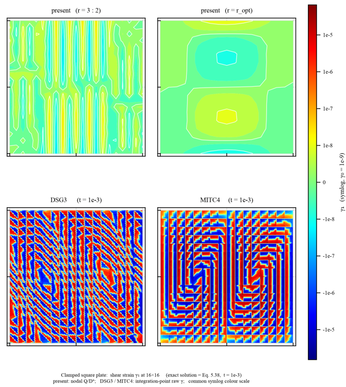
图 4.5 固支方板剪切应变 \gamma_1 的等值线云图 ( 16 \times 16 网格, 统一色标)
