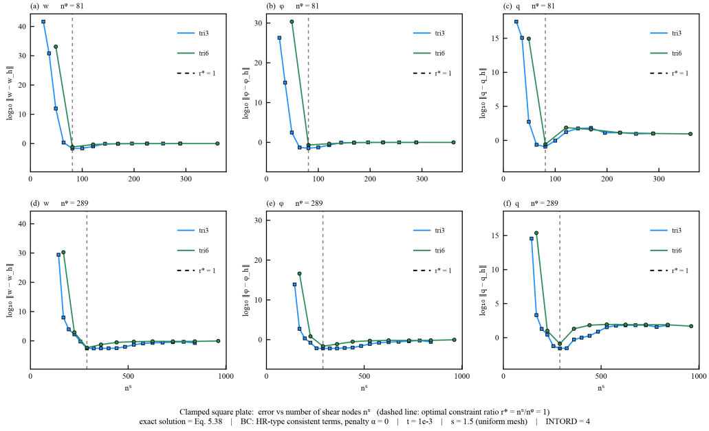
图 4.3 固支方板挠度、转角与剪力误差随剪力节点数的变化（虚线为最优约束比 r^* = 1 ）
