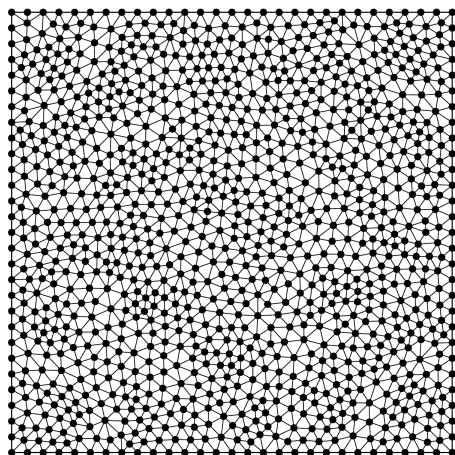
图 4.2 固支方板挠度场的节点布置（图中数字为节点数）
