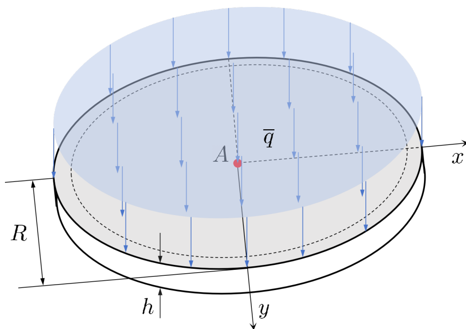
图 4.6 周边固支圆板示意图
