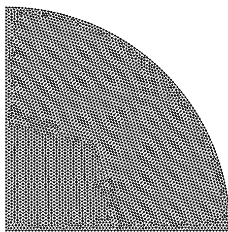
图 4.7 固支圆板挠度场的节点布置 (图中数字为节点数)
