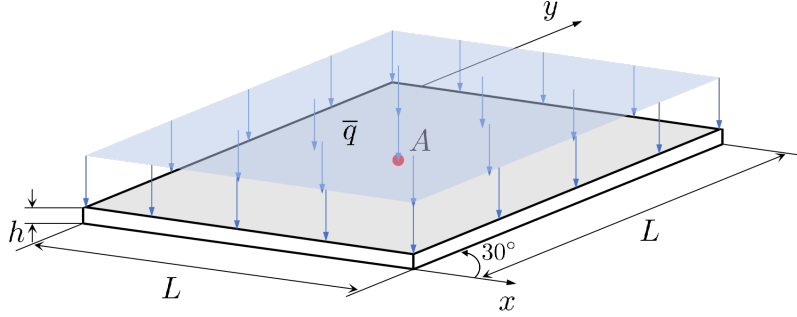
图 4.8 菱形锐角斜板示意图
