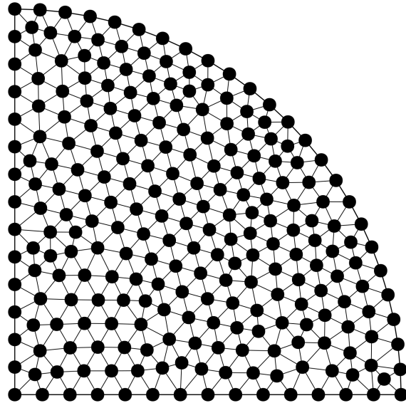
图 4.7 固支圆板问题节点离散
