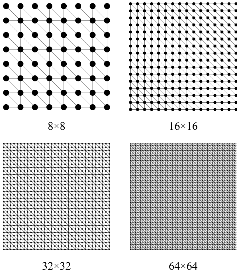
图 4.2 固支方板问题节点离散
