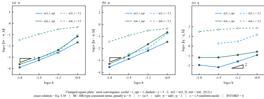
图 4.2 固支方板挠度、转角与剪力误差的收敛曲线（实线为 r = r^* ，虚线为 r = 3:2 ）
