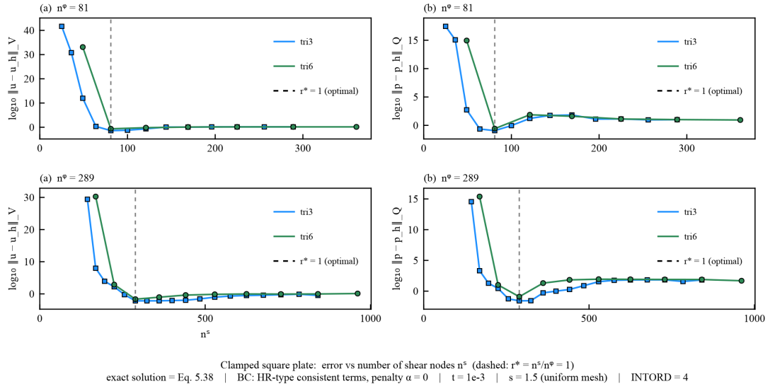
图 4.1 固支方板误差随剪力节点数的变化（虚线为最优约束比 r^* = 1 ）
