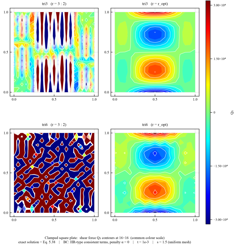
图 4.3 固支方板剪力 Q_1 等值线云图 ( 16 \times 16 网格, 统一色标)
