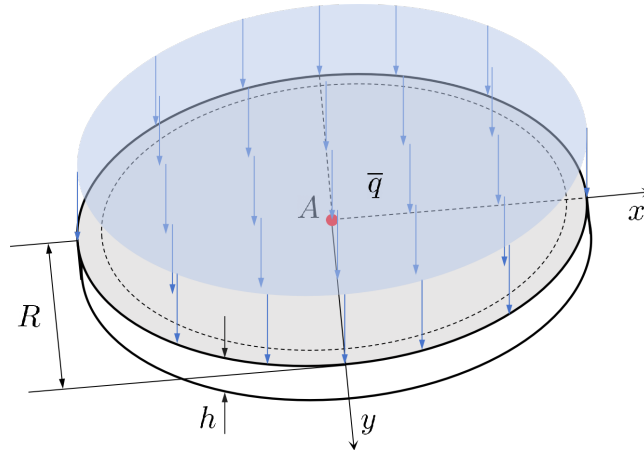
图 4.5 周边固支圆板示意图
