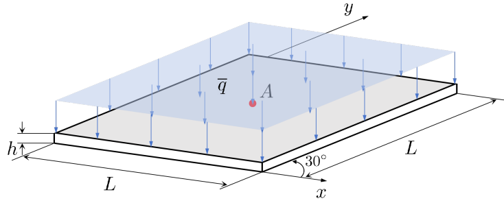
图 4.7 菱形锐角斜板示意图
