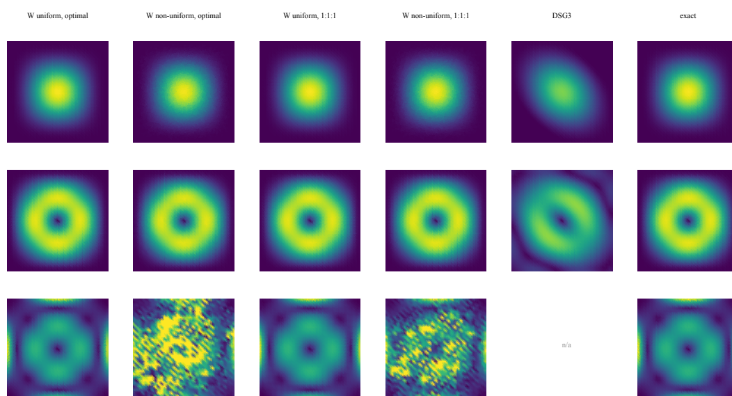
图 4.4 五组 tri3 算例数值解与精确解的云图
