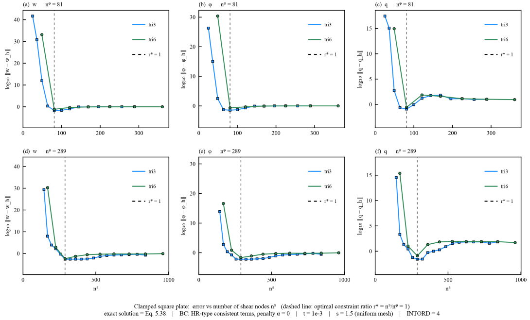
图 4.1 固支方板挠度、转角与剪力误差随剪力节点数的变化（虚线为最优约束比 r^* = 1 ）
