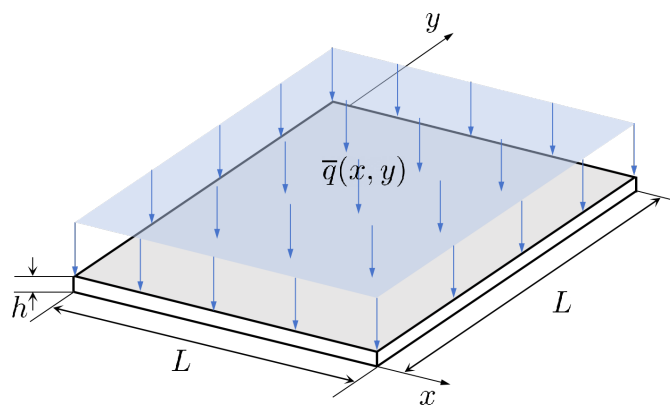
图 4.1 四边固支方板示意图
