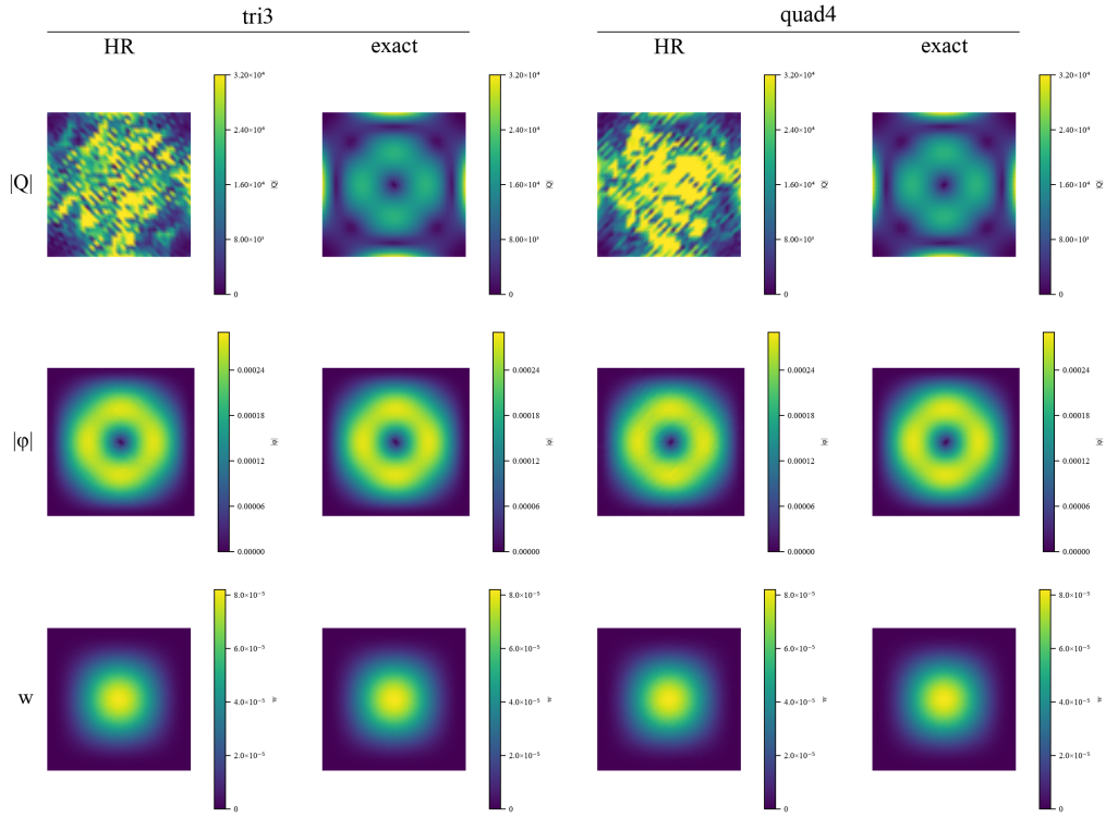
图 4.5 非均匀 W 网格下数值解与精确解的云图对比
