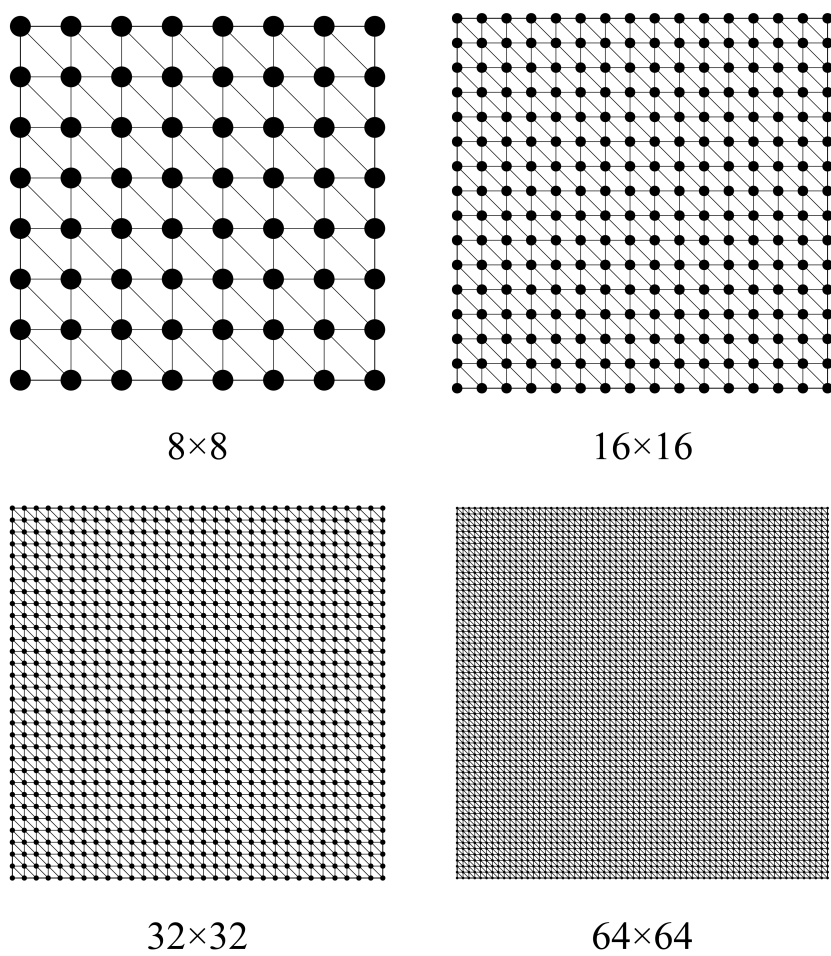
图 4.2 固支方板问题节点离散
