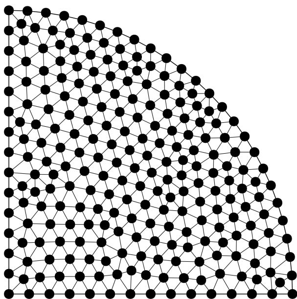
图 4.7 固支圆板问题节点离散
