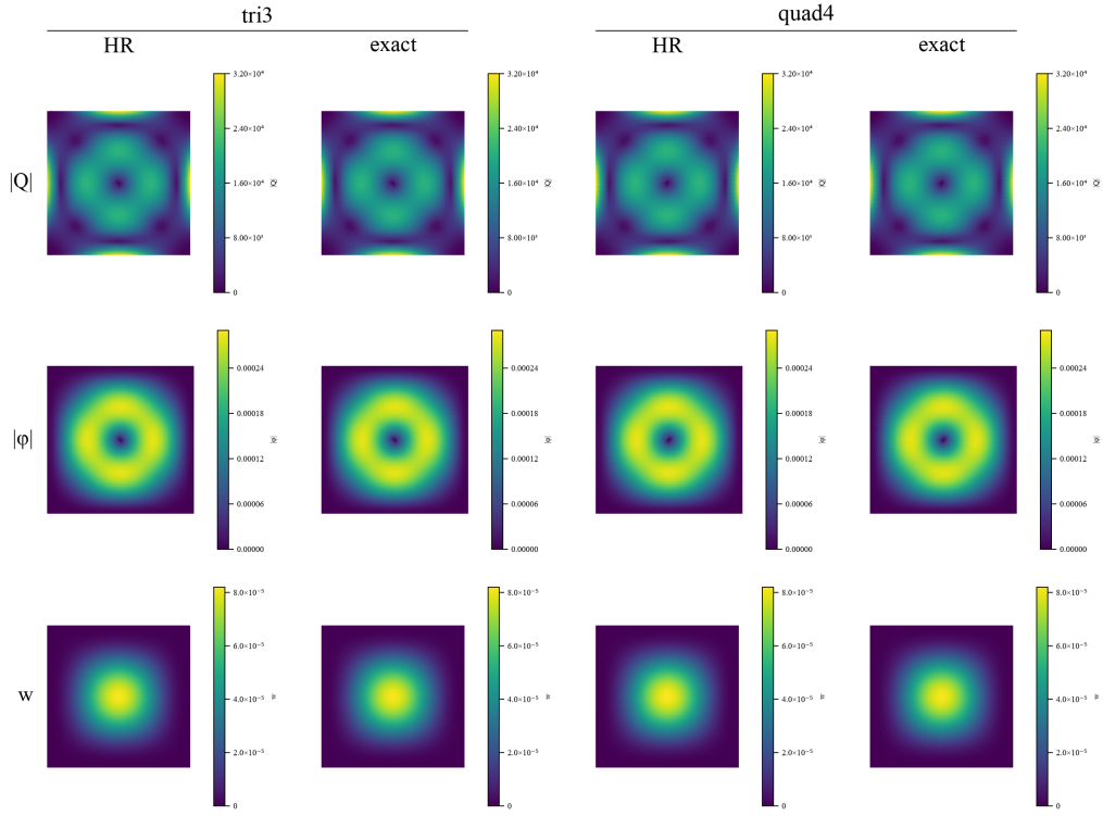
图 4.4 均匀 W 网格下数值解与精确解的云图对比
