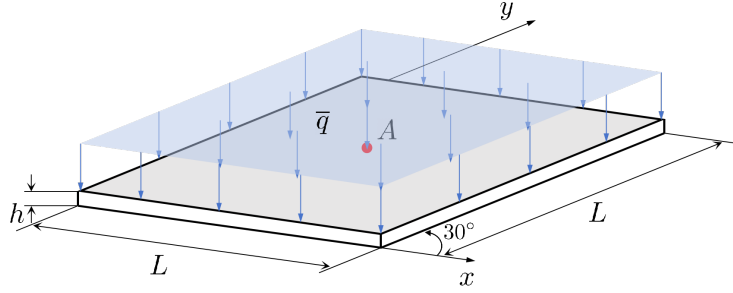
图 4.8 菱形锐角斜板示意图
